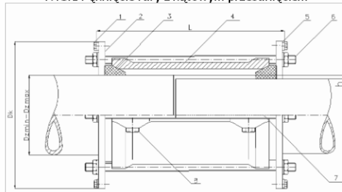
RYS.1 Pęknięcie rury z kątowym przesunięciem
