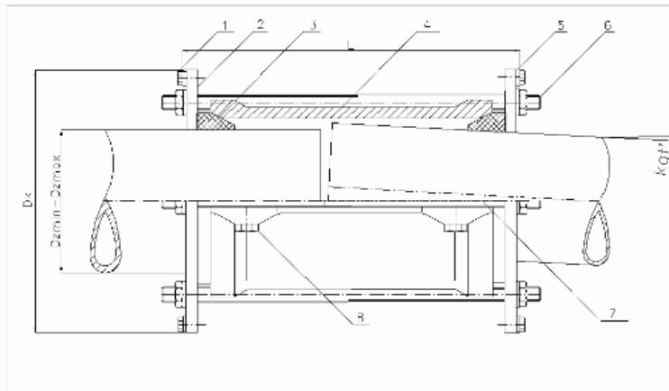
RYS.1 Pęknięcie rury z kątowym przesunięciem
